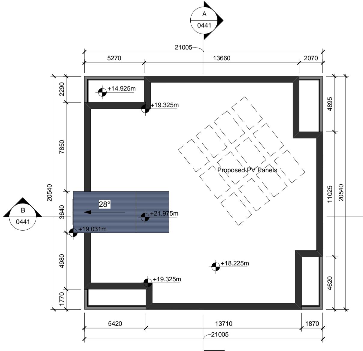
6 Roof Plan 1 : 200
